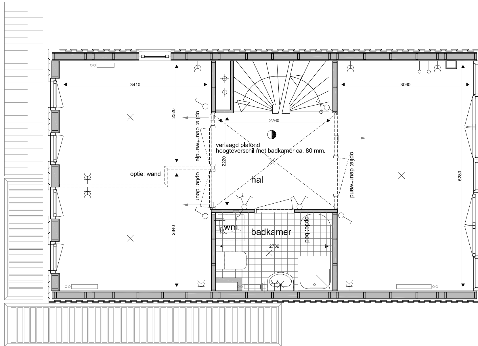
plattegrond 1e verdieping Lakeside P3
