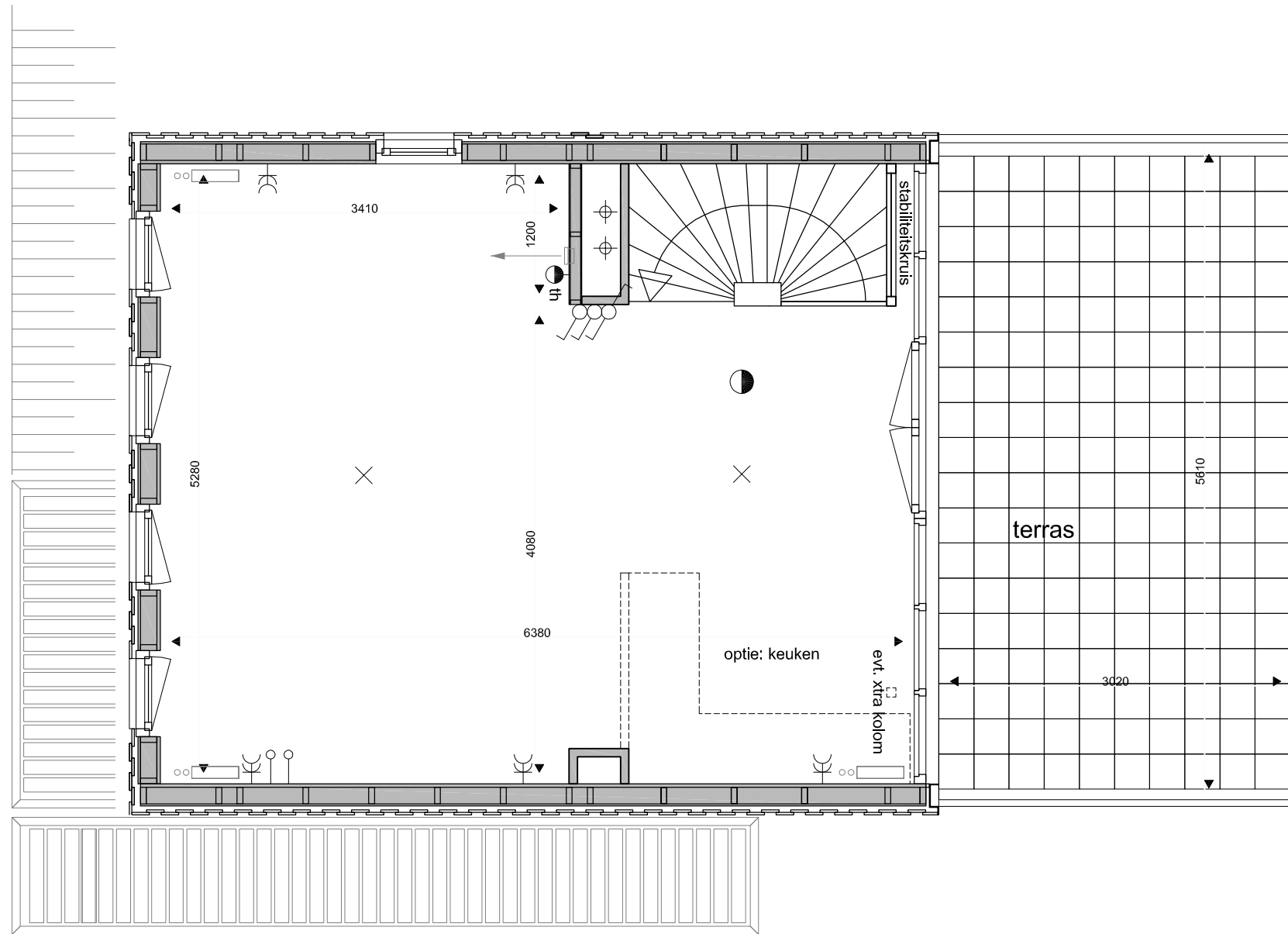
plattegrond 2e verdieping Lakeside P3
