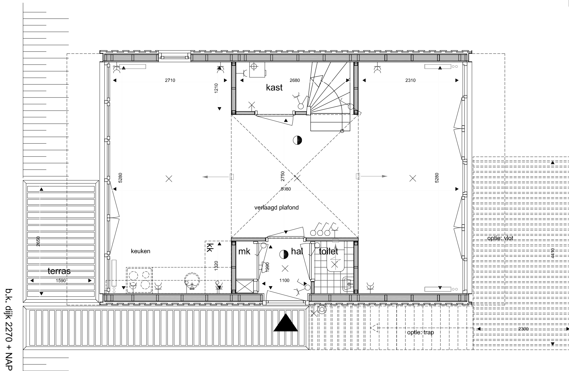
plattegrond begane grond Lakeside P3
