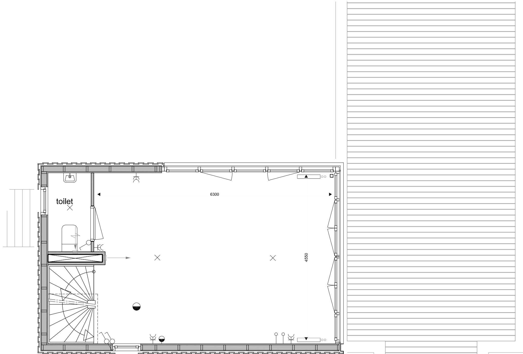
bouwnummer 66 plattegrond 3e verdieping Lighthouse
