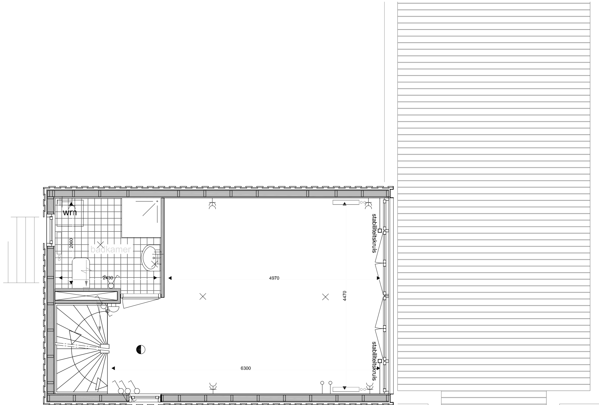
bouwnummer 66 plattegrond 1e verdieping Lighthouse
